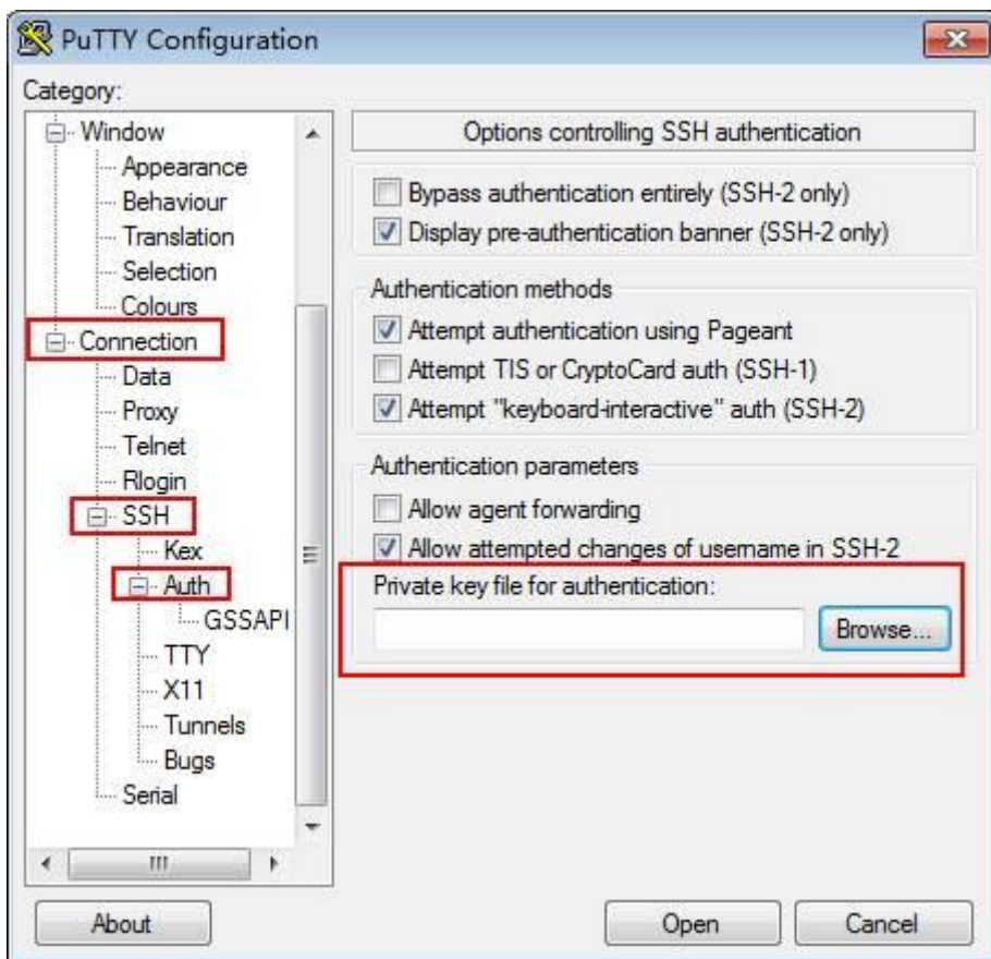
图 7-28 导入私钥
