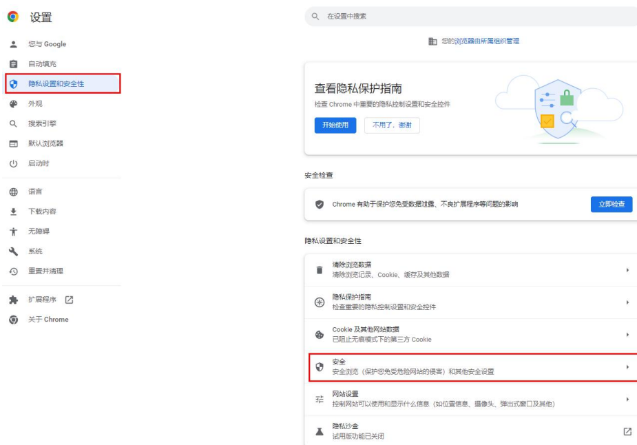
图 7-36 设置页面
