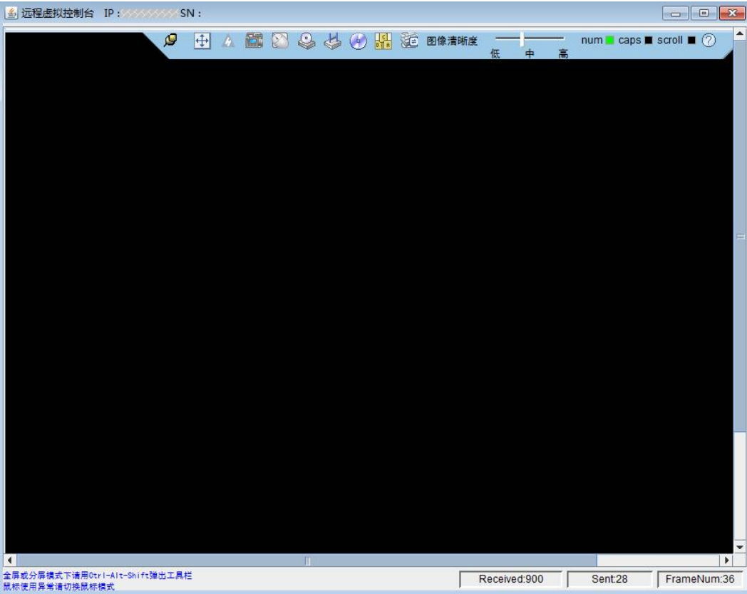
图 5-81 Java KVM
