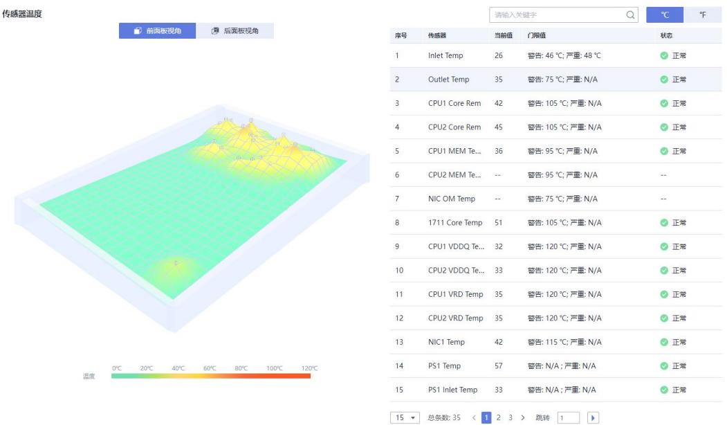
图 5-28 传感器温度
