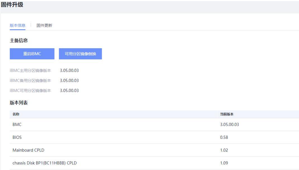
图 5-63 固件升级
