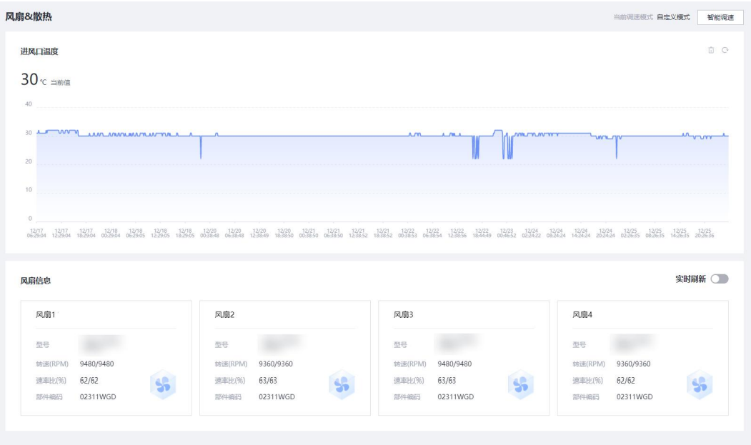
图 5-27 风扇&散热
