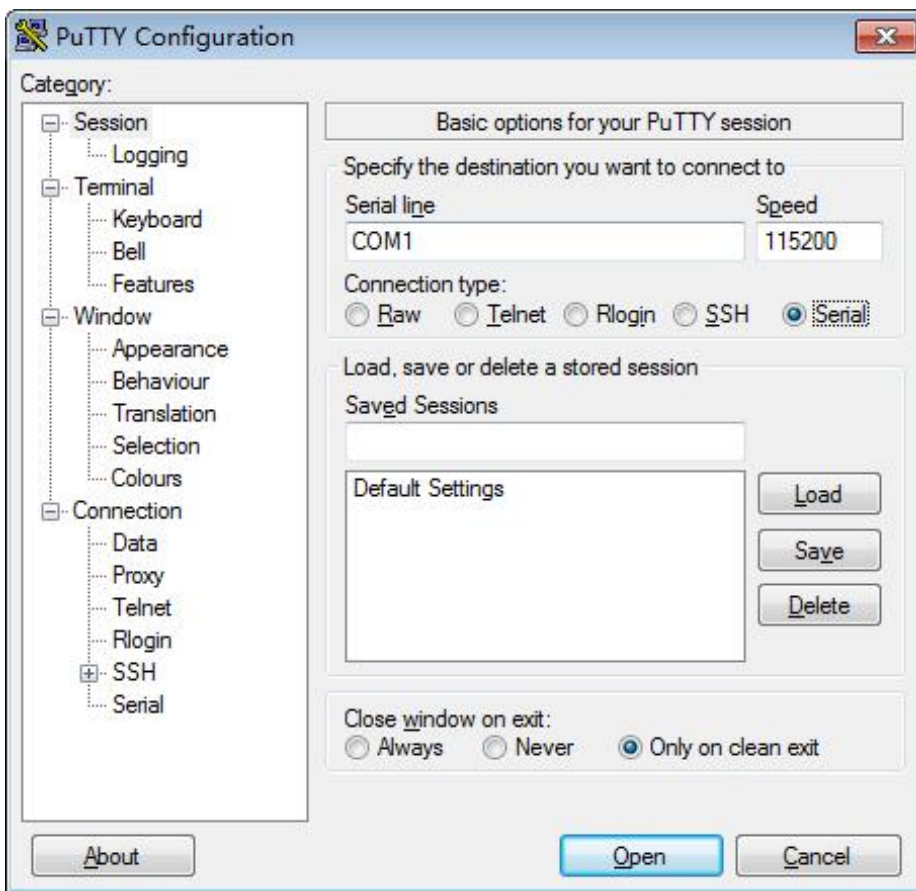
图 7-1 PuTTY Configuration
