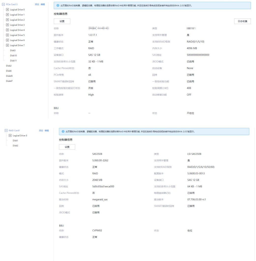
图 5-13 存储管理
