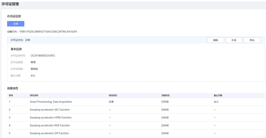
图 5-68 许可证管理
