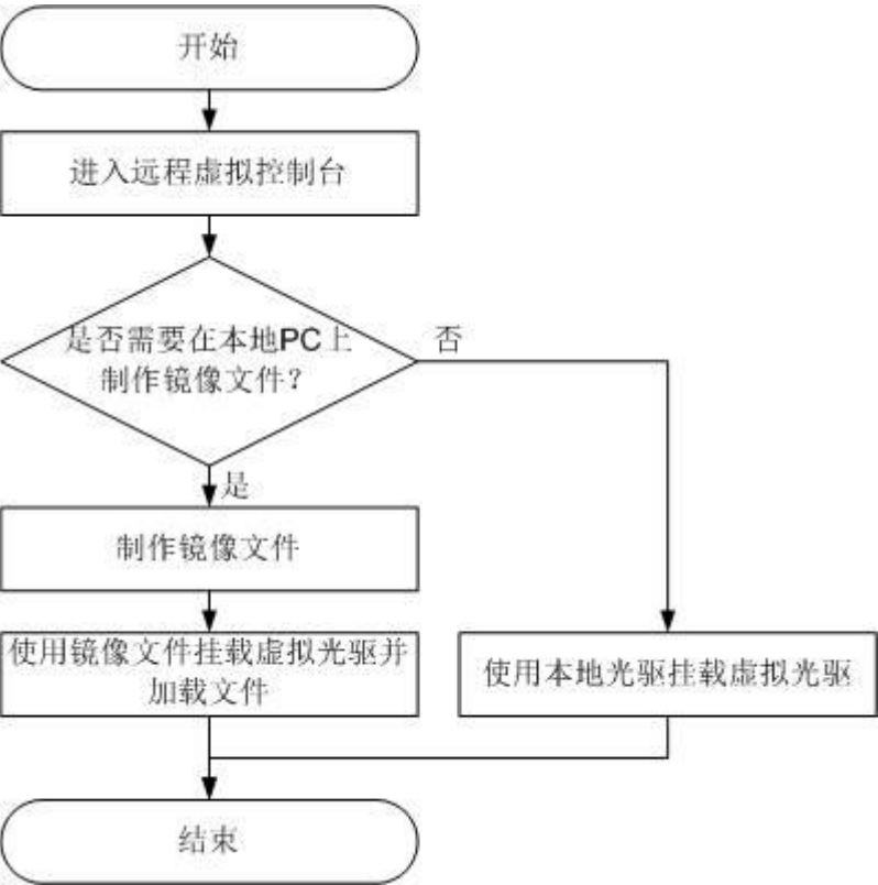
图 5-80 使用流程
