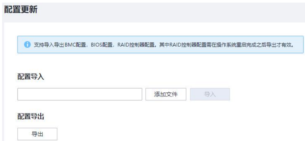
图 5-64 配置更新
