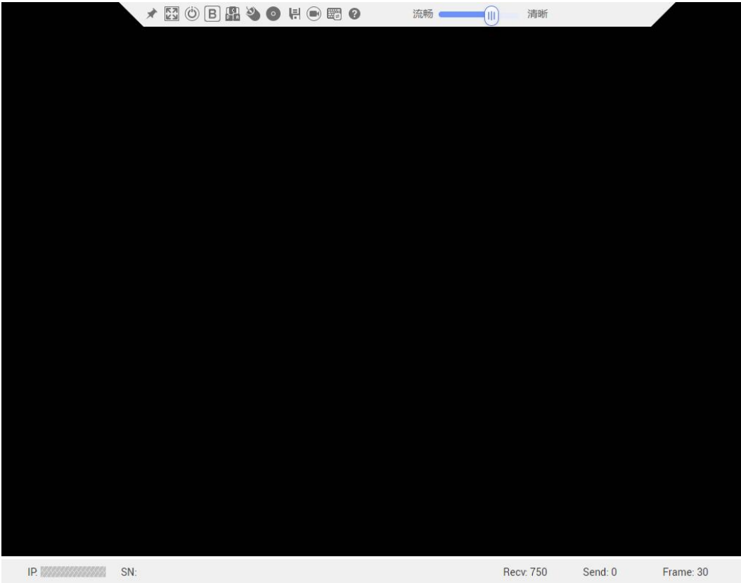
图 5-73 HTML5 KVM
