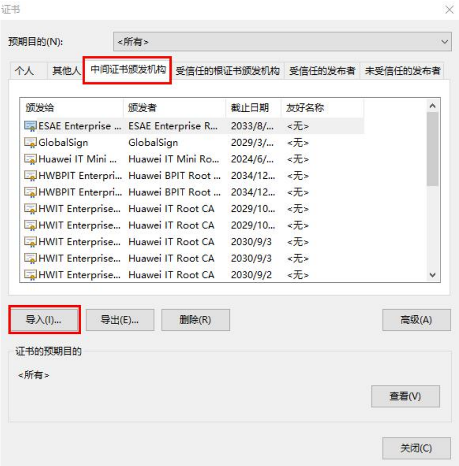
图 7-38 证书窗口
