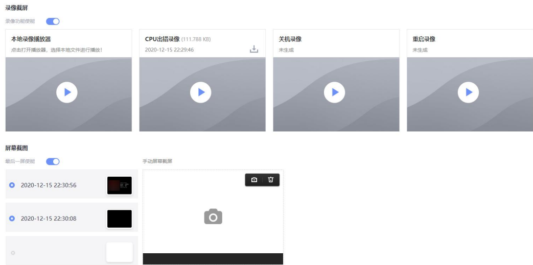
图 5-35 录像截屏
