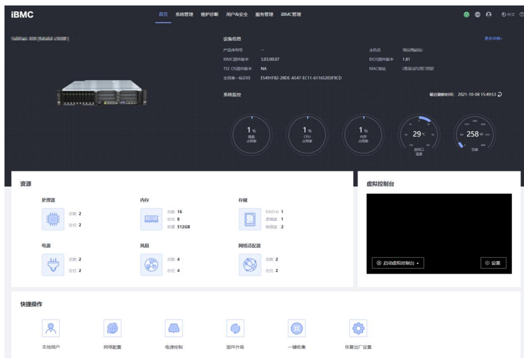
图 5-4 首页
